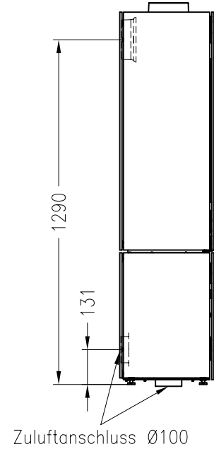
Seitenansicht von links M~1:20
