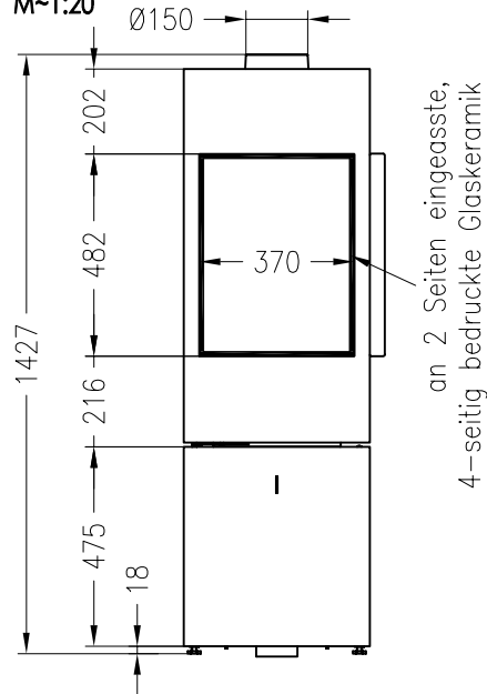
Vorderansicht M~1:20
