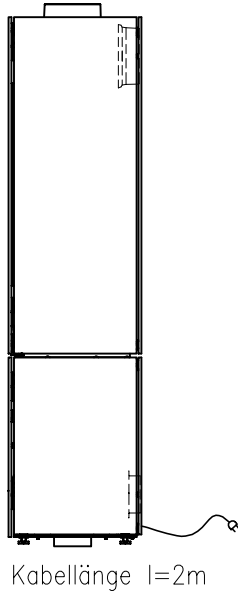
Seitenansicht von rechts M~1:20
