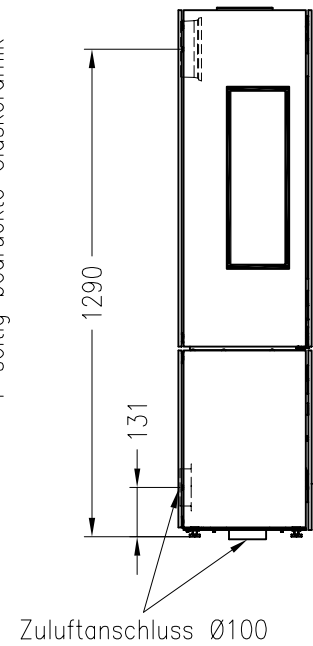
Seitenansicht von links M~1:20
