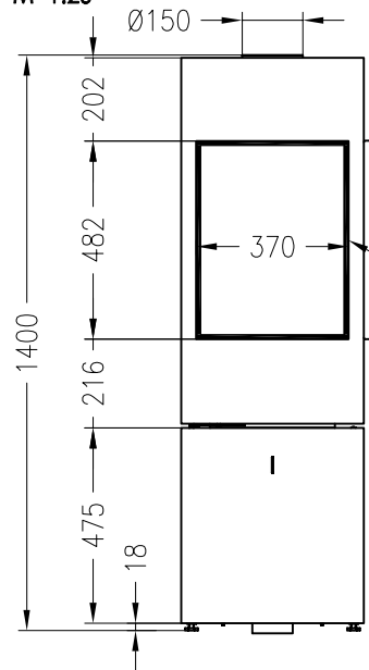
Vorderansicht M~1:20
