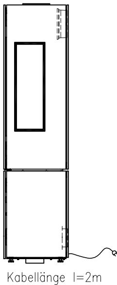
Seitenansicht von rechts M~1:20
