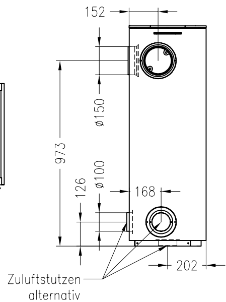
Rückansicht M~1:20
