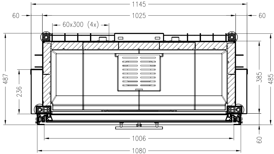
Horizontalschnitt M~1:10
